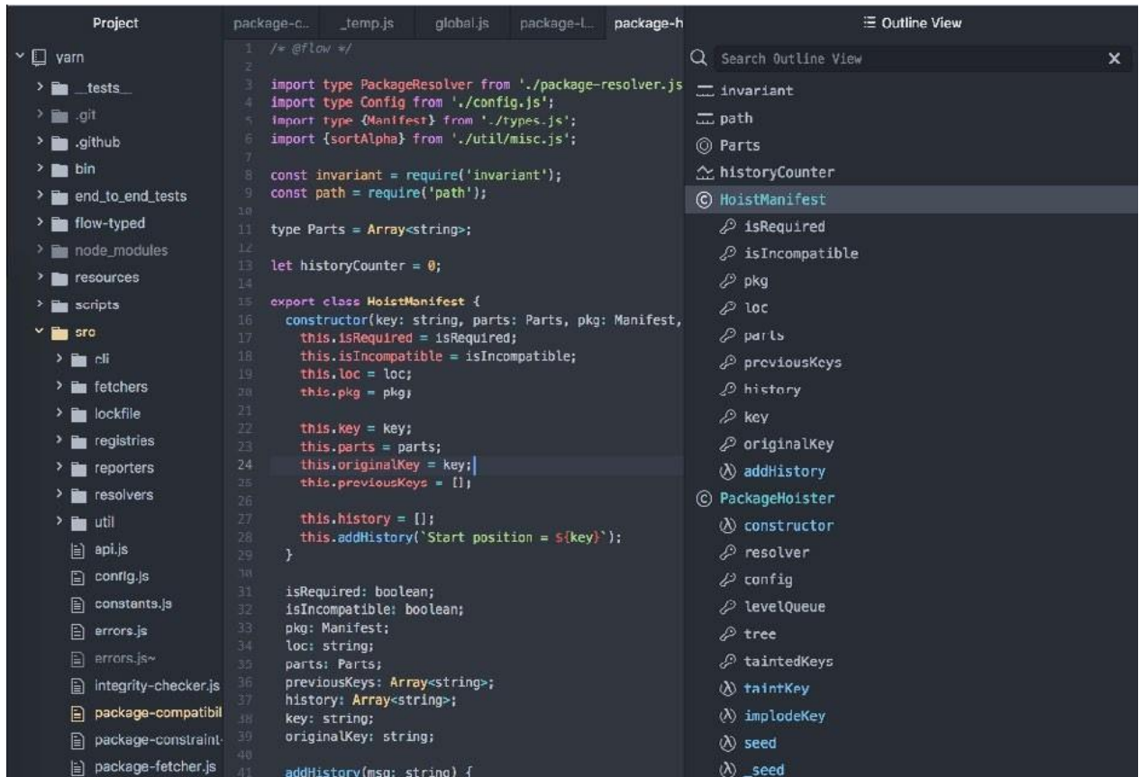
Рис. 9. Интерфейс Atom
