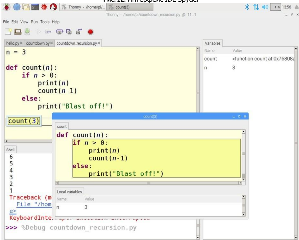
Рис. 13. Интерфейс IDE Thonny
