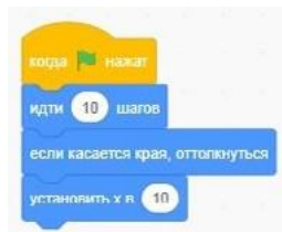
Рис. 5. Фрагмент программы в среде Scratch
