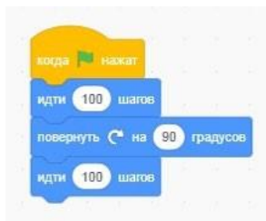
Рис. 86. Вид программы в среде Scratch
