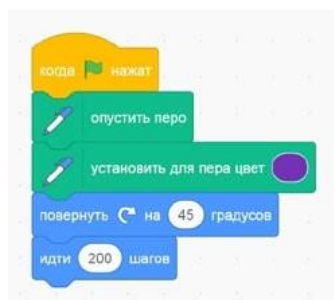
Рис. 165. Вид скрипта в среде Scratch
