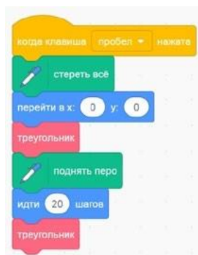
Рис. 149. Вид программы с новым блоком
